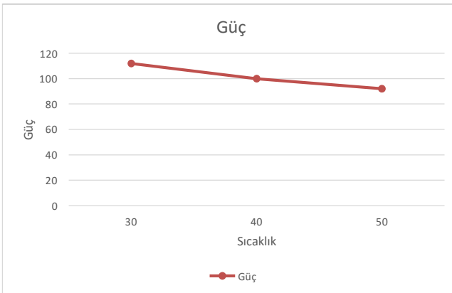
Sıcaklığa Bağlı Güç Değişimi
