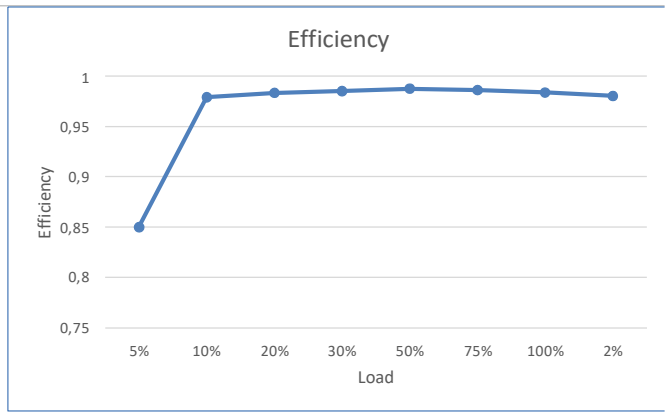
Verimlilik Eğrisi
